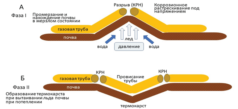
Рис. 8 / Fig. 8. Коррозионные риски: (А) при промерзании и нахождении почвы в мёрзлом состоянии, (Б) при вытаивании льда и формировании термокарста при потеплении / Corrosion risks: (A) when freezing and the soil is in a frozen state, (B) when ice melts and thermokarst forms during warming
