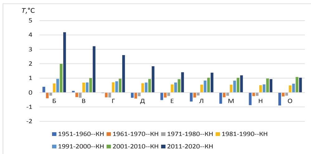
Рис. 2 / Fig. 2. Изменение среднегодовой температуры воздуха относительно климатической нормы (КН), °C / Change in the average annual air temperature relative to the climatic norm (CN), °C
